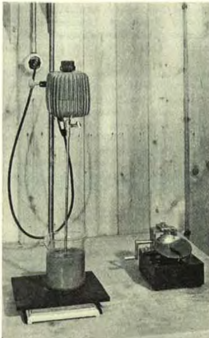
Bild 8. Links Vibromischer zur Aufbereitung von Suspensionen; rechts Casagrande-Apparat zur Bestimmung der Fließgrenze bindiger Materialien
